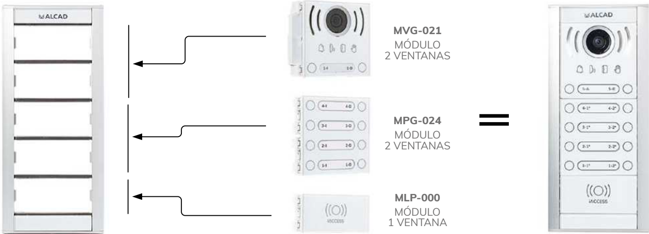
FRA-005 BASTIDOR 5 VENTANAS
