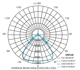
90° Lente de ángulo apertura Beam angle lens Lente de ângulo de abertura
