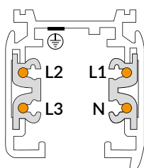
VISTA FRONTAL ORIENTACIÓN NEUTRO DERECHA CONEXIÓN CON R
