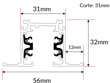
VISTA FRONTAL ORIENTACIÓN NEUTRO IZQUIERDA CONEXIÓN CON L
