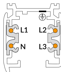
VISTA FRONTAL ORIENTACIÓN NEUTRO IZQUIERDA CONEXIÓN CON L
