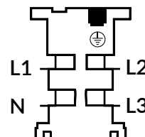
CONECTOR INICIAL VISTA FRONTAL NEUTRO IZQUIERDA TRCK-038/037
