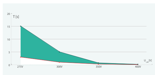
Curva de tensión / tiempo según normativa UNE-EN-50550
